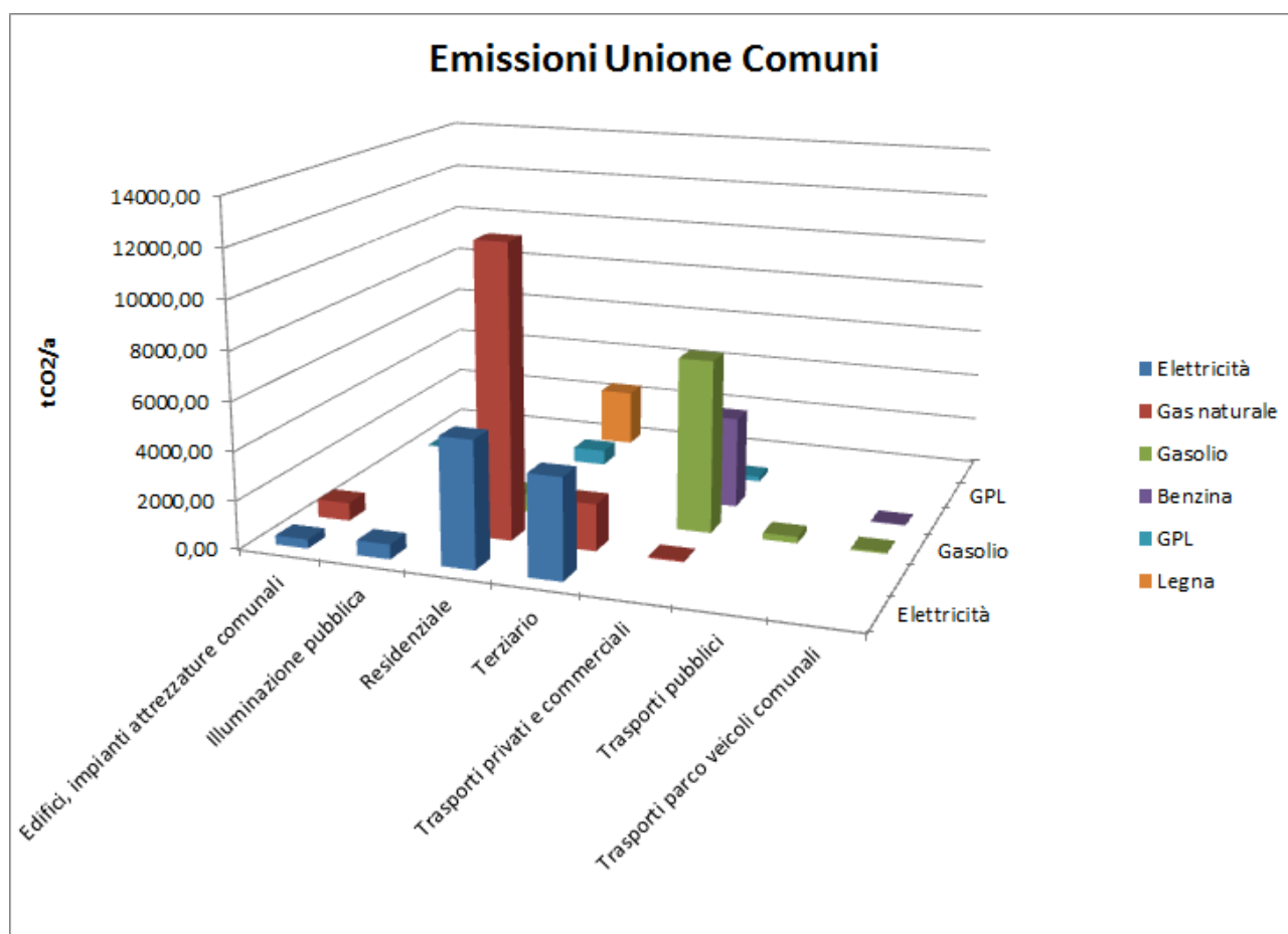
Figura – Emissioni di CO2 suddivisi per fonte di energia e per settore nei territori comunali dell’Unione dei Comuni delle Valli Antigorio, Divedro e Formazza
