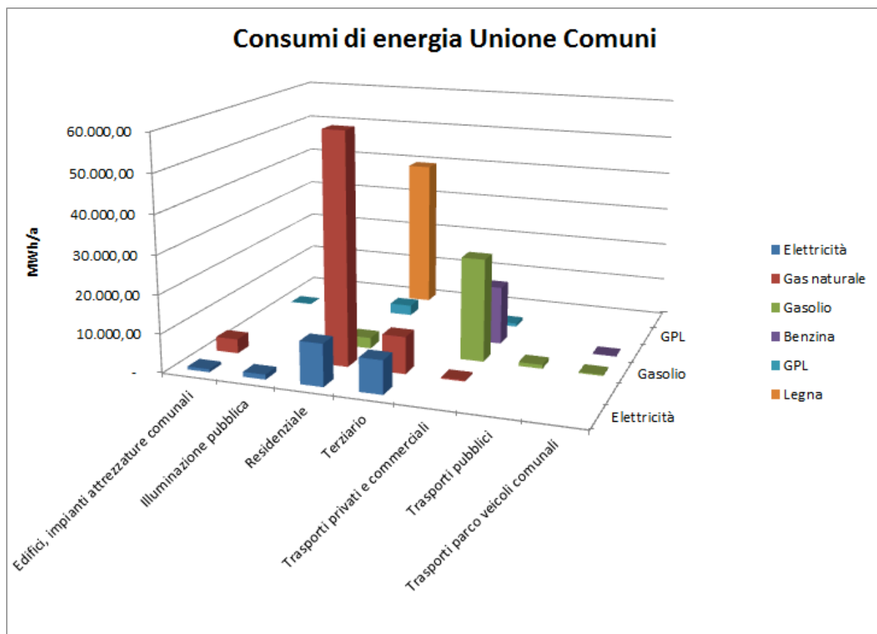
Figura – Consumi di energia suddivisi fonte e per settore nei territori comunali dell’Unione dei Comuni delle Valli Antigorio, Divedro e Formazza
